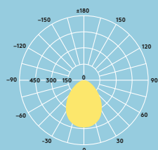
Przełącznik strumienia światła @ Anna Vario Flex
